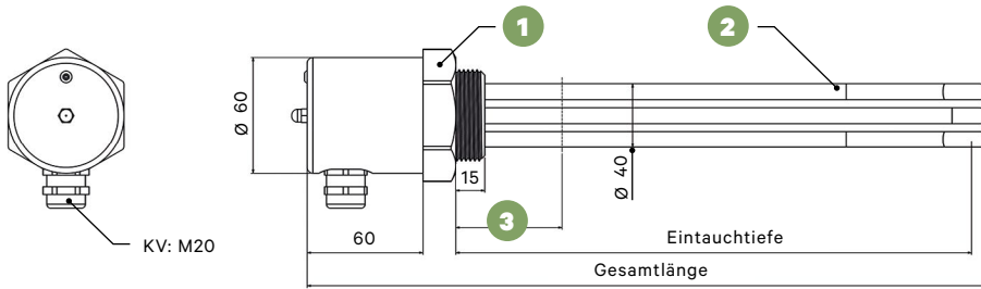
Einschraubheizkörper ohne Temperaturregler
