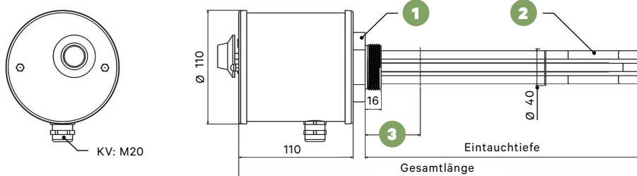
Einschraubheizkörper inkl. Temperaturregler/-begrenzer
